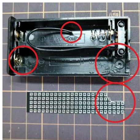
基板カット、ケース加工
