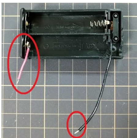
リード線半田付け
