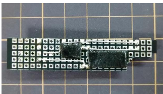
基板半田付け（裏）
